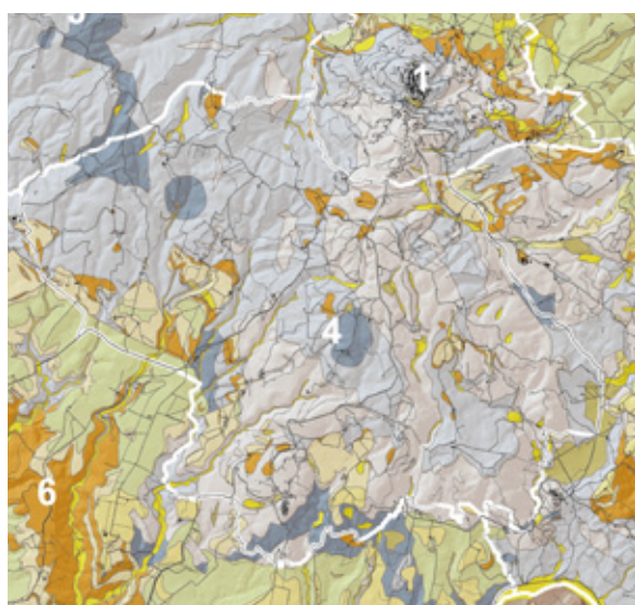
Carta litotecnica
