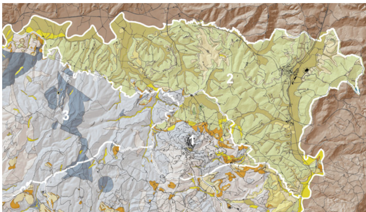
Carta litotecnica
