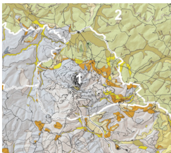
Carta litotecnica
