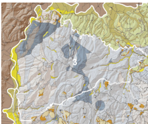
Carta litotecnica
