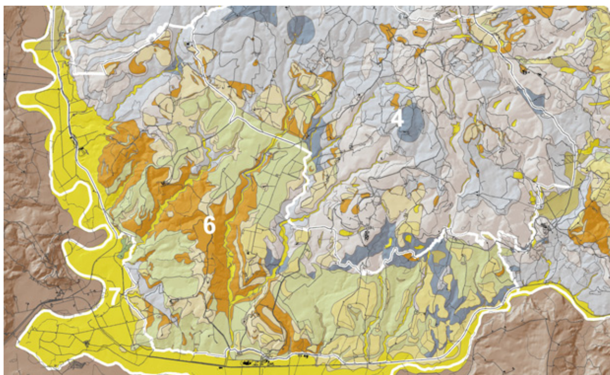
Carta litotecnica
